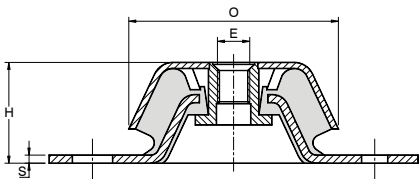
Antivibrante a campana rettangolare zincata bianca.
